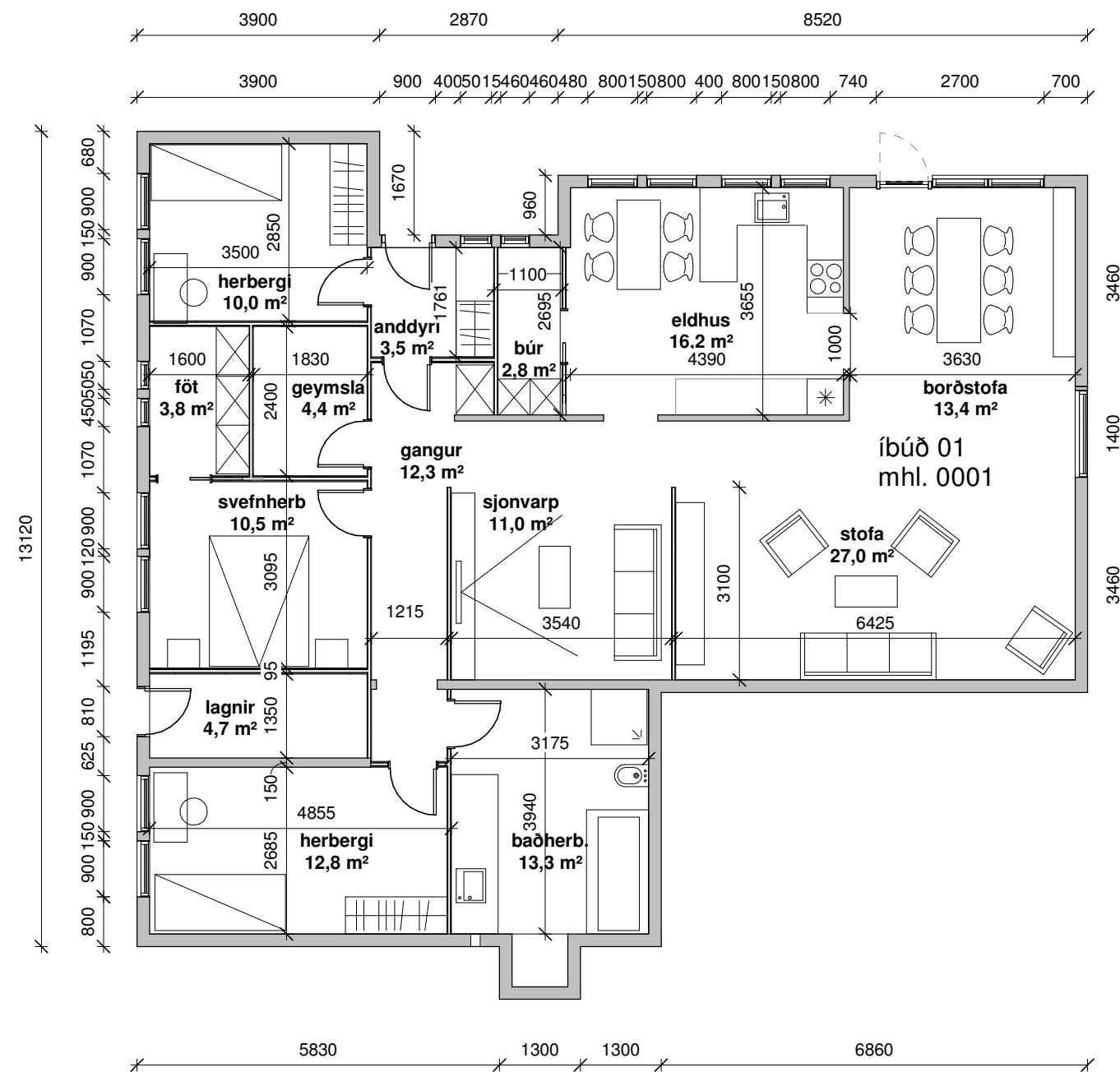
1. HÆÐ 1 : 100
