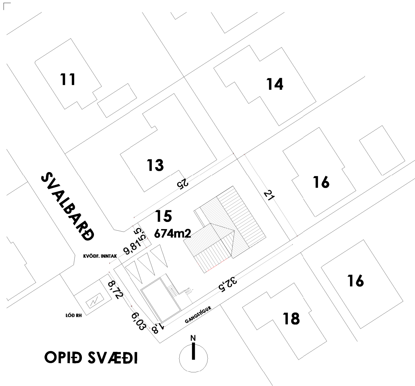
0. AFSTÖÐUMYND/LÓÐ 1 : 500
